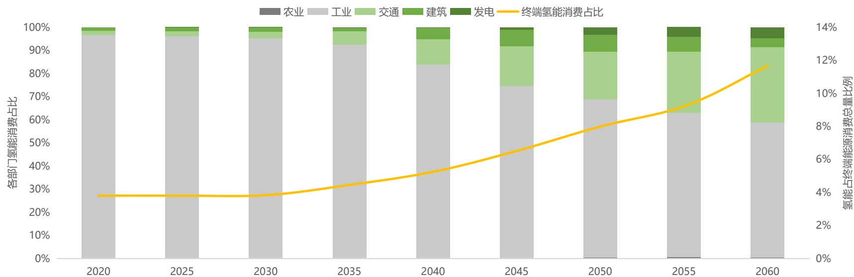
我国氢能多元化应用预测
