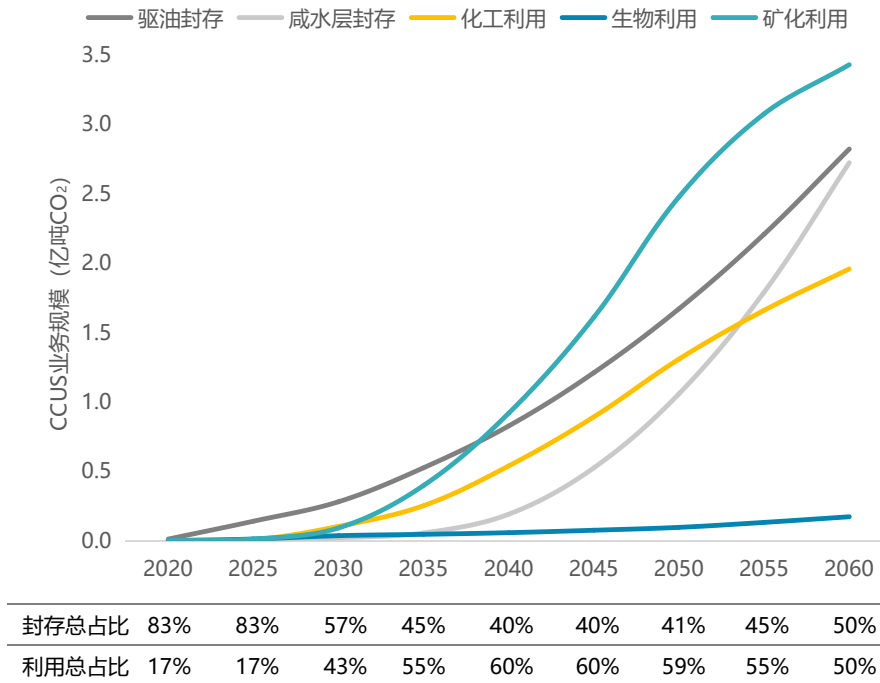
我国各CCUS业务路径发展规模预测
